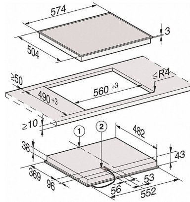
KM 6520 FR, KM 6538 FR (skitse)
